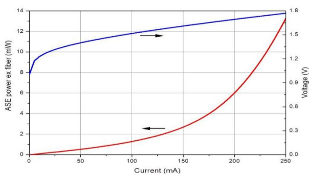
L-I-V 曲线
