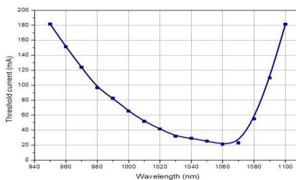
阈值电流
