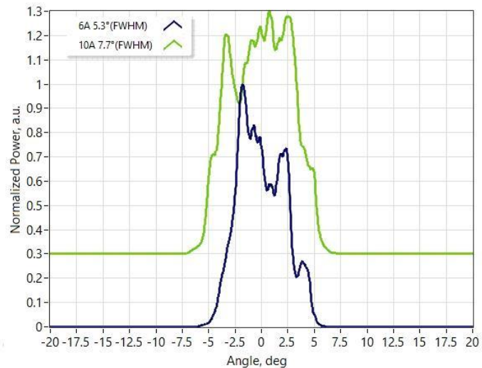
慢轴远场
