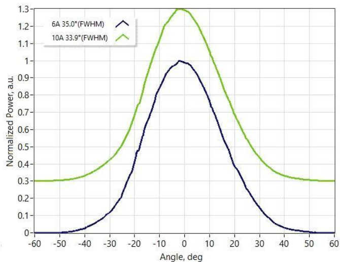
快轴远场
