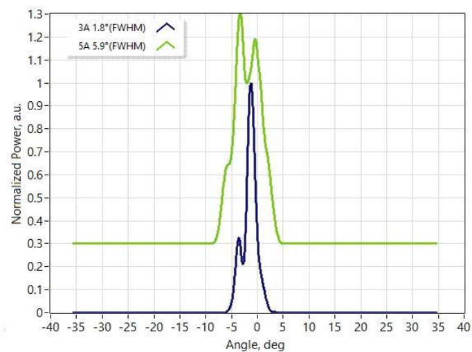
慢轴远场
