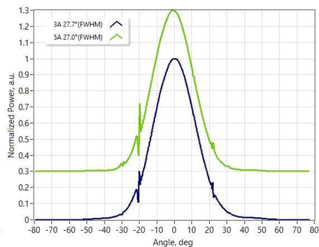
快轴远场
