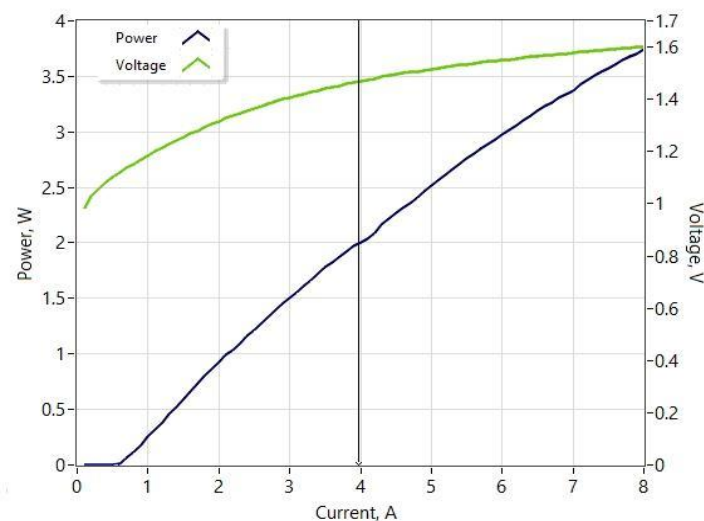
光-电流-电压特性
